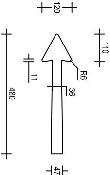
W8-3L(C) 900 x 600
