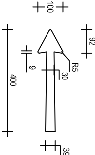
W8-3L(B) 750 x 500
